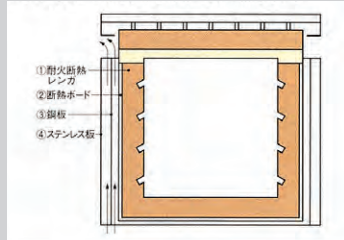
DAM シリーズの構造図
