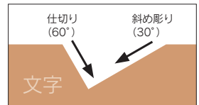
図c 片切り彫り 切り出して仕切り(約60°)を入れ、逆方向から丸刀などで斜め(約30°)に彫る。
